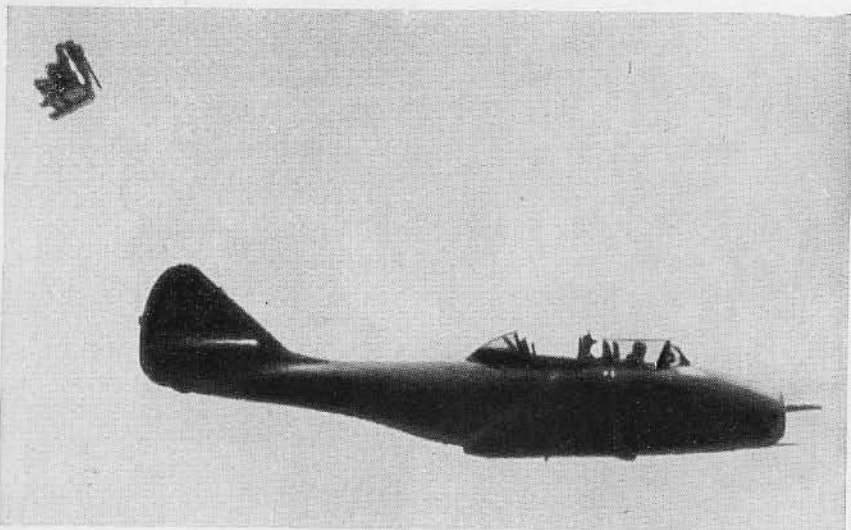
МиГ-9 УТИ. Летчик-испытатель М. Л. Галлай сбрасывает катапультируемое кресло с манекеном.
